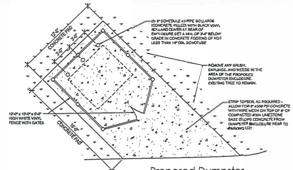
2 Enclos SCALE: 1/4" = 1'-0"
